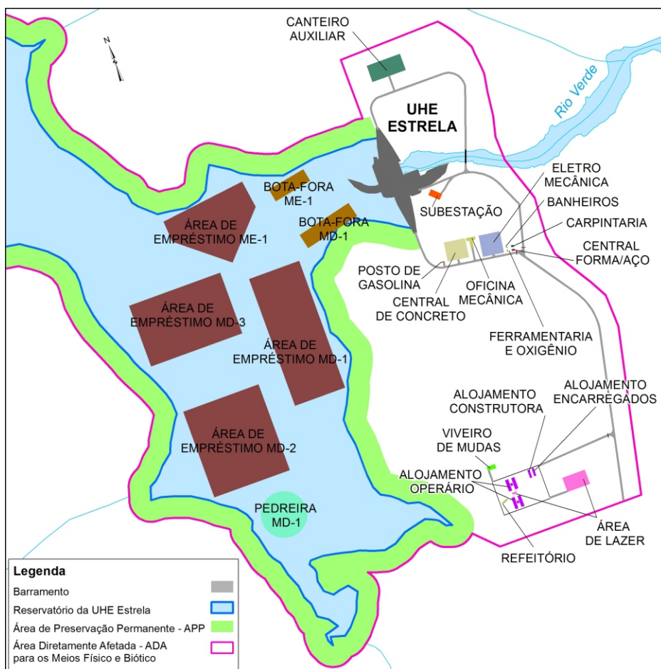
Arranjo geral da área de implantação da barragem
